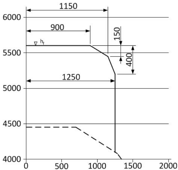
Figur 3: NO1-referanseprofil for pantograf
