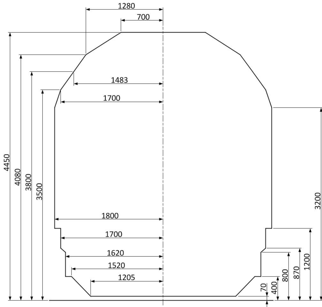
Figur 1: Referanseprofil for dynamisk mål NO1
