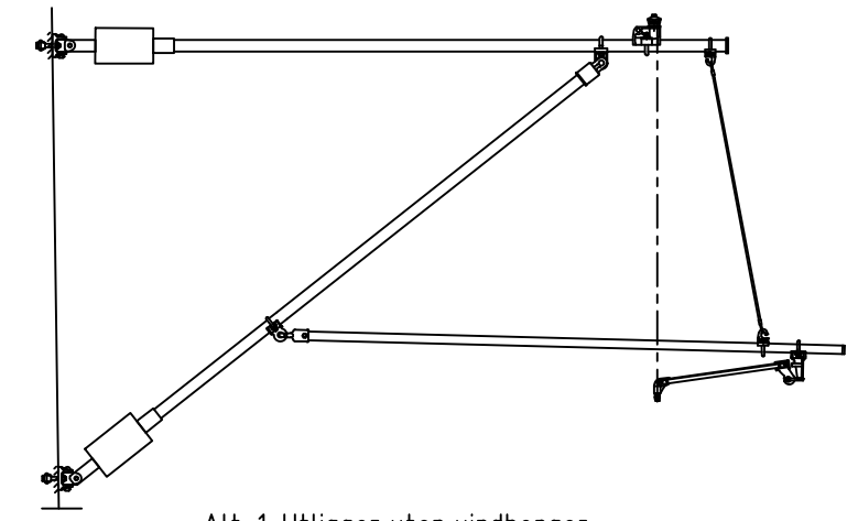
Alt. 1: Utligger uten vindhenger. Pos. 14 og 15 utgår.
