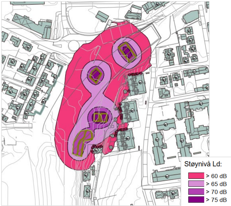
Figur 2. Støykart jetpeling for byggegrøp Kransen Øst.
