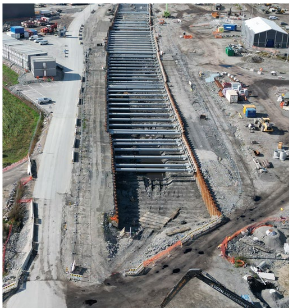
Figur 2. Bilde fra utgravingen av kulvert Carlberg, hvor det er etablert avstivningsrør. Tilsvarende utgraving og avstiving skal gjøres for kulvert Larkollveien.
