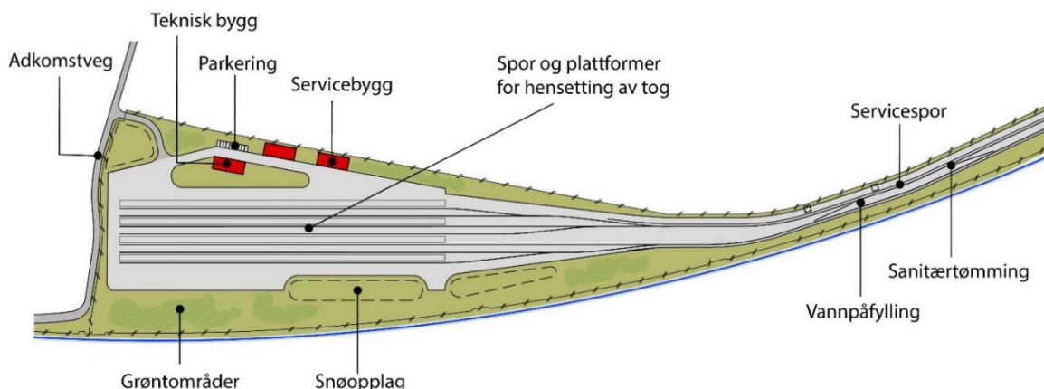
Figur 3.1 Prinsippsskisse av et hensettingsanlegg. Plassering av- og antall spor, bygg og servicefasiliteter i dette prosjektet vil avvike fra figuren
