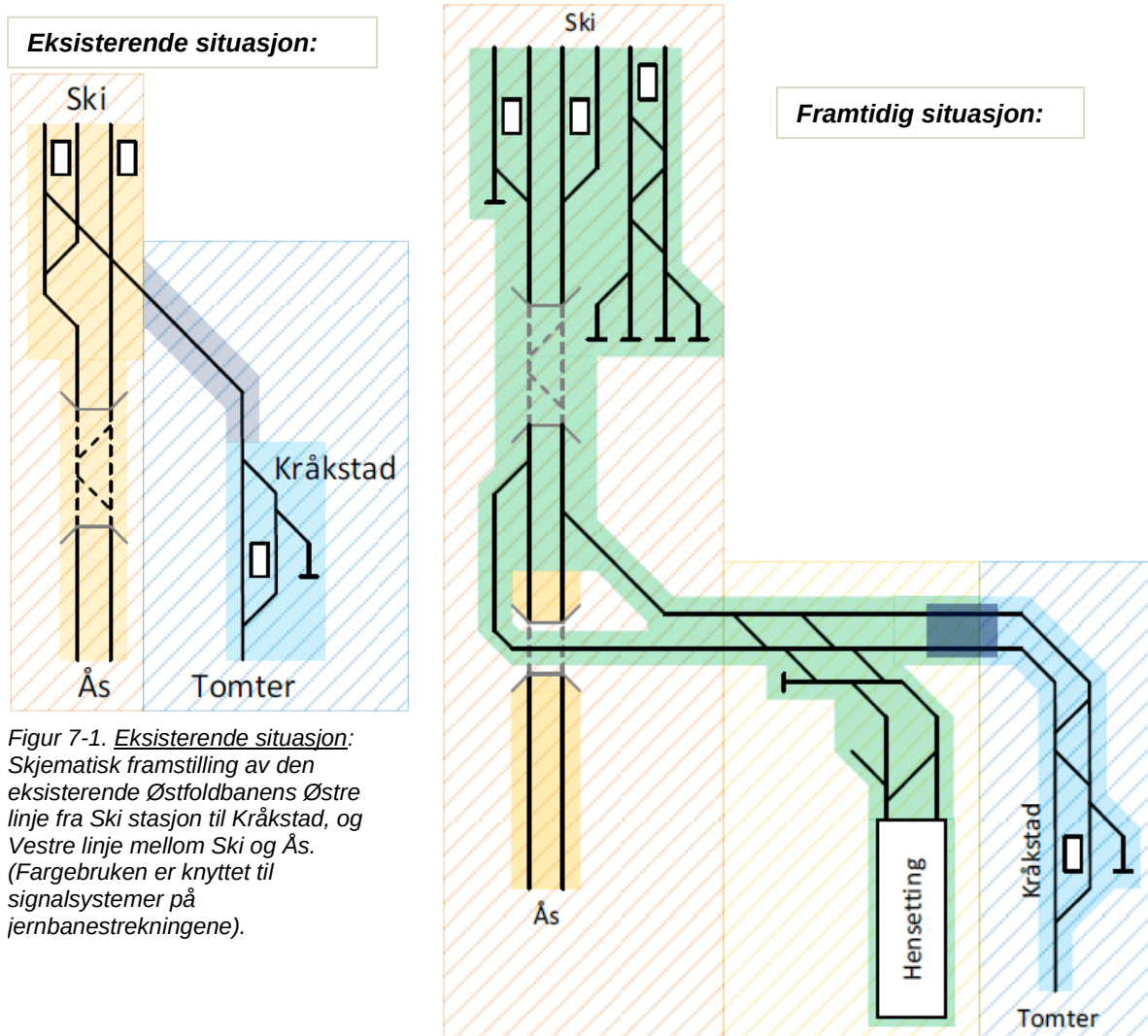
Figur 7-2: Framtidig situasjon: Skjematisk framstilling av ny avgrening av Østfoldbanens Østre linje. Det etableres ny avgrening fra Vestre linje sør for Ski stasjon til Kråkstad, med påkobling til nytt anlegg for togparkering/hensetting. Ski stasjon bygges om i sammenheng med etablering av Follobanen. (Fargebruken er knyttet til signalsystemer på jernbanestrekningene).
