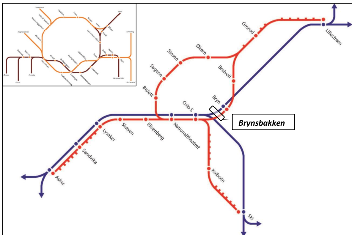
Figur 3-1 KVV Oslo-navet anbefaler blant annet ny jernbanetunnel og metrotunnel gjennom Oslo sentrum. Illustrasjonen viser prinsipp for separering av togtrafikken. Regiontog benytter det blå systemet og S-bane (utvikling av lokaltog) det røde. Innfelt øverst til venstre er anbefalt prinsipp for metrosystemet. (Kilde: KVV Oslo-navet). Tiltak i Brynsbakken regnes som en forutsetning for ny jernbanetunnel (Brynsbakkens beliggenhet er markert på figuren).
