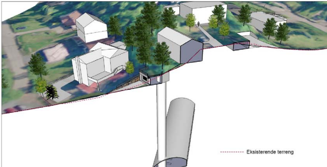
Illustrasjonen viser snitt/oppriss/perspektiv av rømningsrommet ved Njålveien 24.
